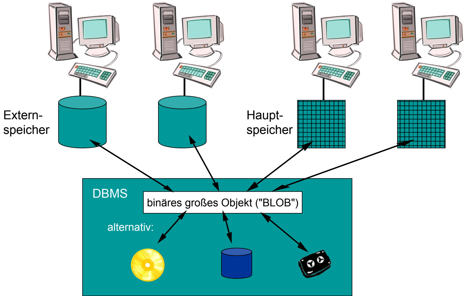
Bild 13.1 Speichergeräte-Unabhängigkeit
